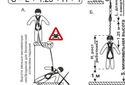
Рис. 6. Расчет высоты свободного пространства под пользователем массой 100 кг для безопасной остановки падения
