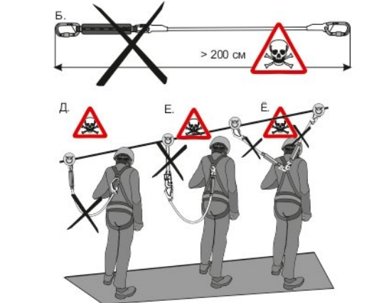
Рис. 7. Использование амортизатора совместно с СИЗ ползункового типа на гибкой анкерной линии
