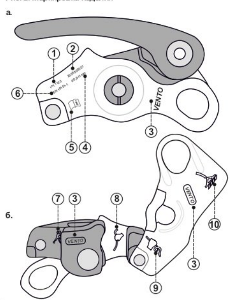
Рис. 2. Маркировка изделия
