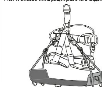
Рис. 4. Способ интеграции рабочего сиденья
