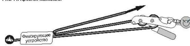
Рис. 14. Простой полиспаст
