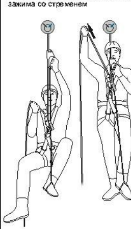
Рис. 13. Подъем с использованием зажима со стреленом
