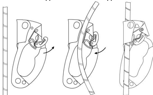
Рис. 3. Укладка веревки в зажим
